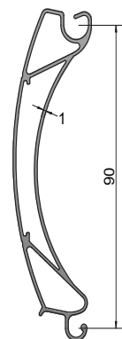
LÂMINA DUPLA (ALUMÍNIO) 0,784 Kg/m
